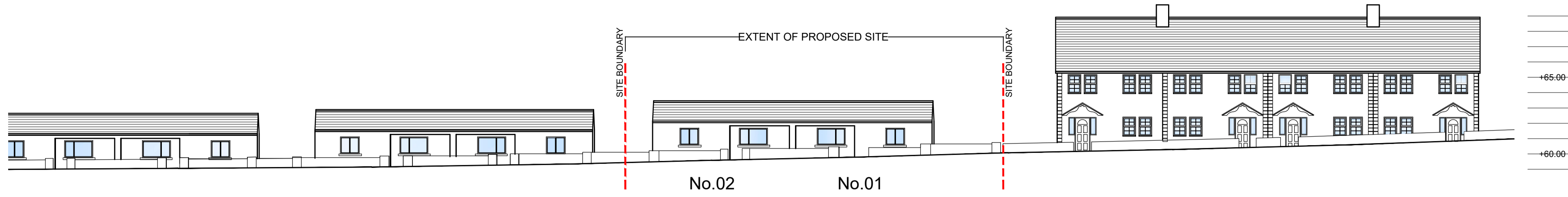
1 GREEN RD .ELEVATION Scale: 1:200@A1
